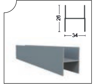
YNSRM-1009 Birleştirme Adaptörü Joining Adapter
