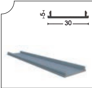
YNSRM-1010 Dikme Kapama Çatısı Side Cover Profile
