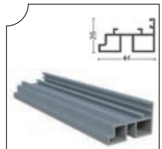
PRGLD-1006 Tıjlı Kollu Fıtil Karşılığı Espagnolette Arm Opposite Seal
