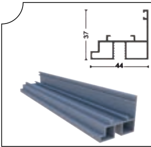
PRGLD-1009 İspanyolet Kol Profil Karşılığı 8 mm Espagnolette Arm Profile Of Opposite
