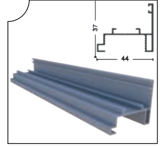
ISICM31-1017 İspanyolet Kollu Profil Espagnolette Arm Profile Of Opposite
