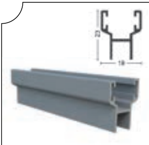
ALMFTL-1002 Büyük H Fıtil Big H Seal
