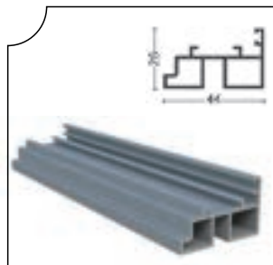
PRGLD-1006 Tıjlı Kollu Fitil Karşılığı Ağırılık/Weight Espagnolette Arm Opposite Seal 0.61 kg/m
