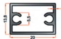
Orta Kayıt Profili Meeting Rail Profile
