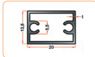
Lüks Kapi Orta Kayıt Profili Luxury Door Meeting Rail Profile
